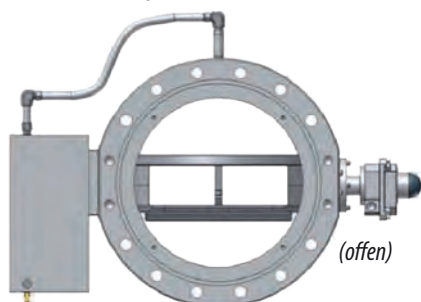
BPIV™ gegendruckunabhängige Knickstab-Druckentlastung
